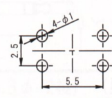
基板取付穴寸法参考図 (t1.6)
