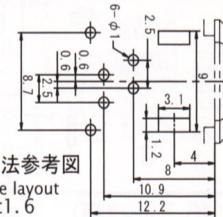
基板取付穴寸法参考図 (t1.6)
