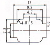
パネル取付穴寸法参考図 適合シャーシ厚 t1.6
