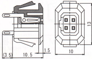
パネル取付穴寸法参考図 適合シャーシ厚 t1.6
